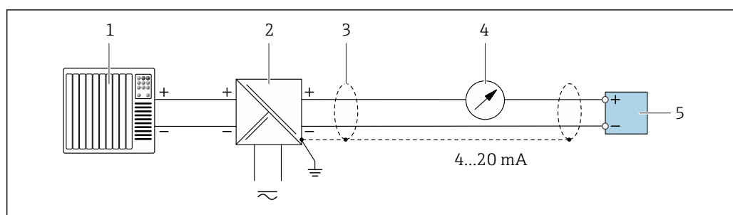
8 Пример подключения для токового выхода 4...20 мА HART (пассивного)
