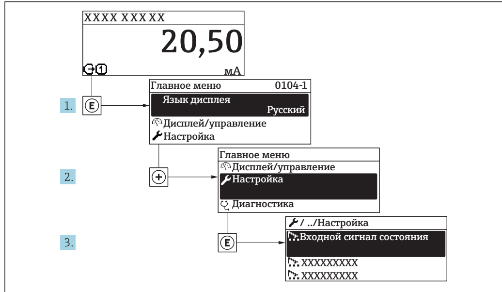
25 Пример индикации на локальном дисплее
