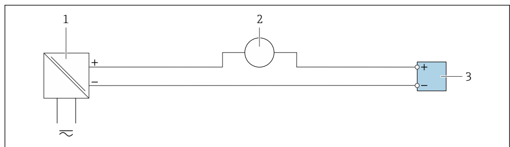
17 Пример подключения для точкового входа 4...20 мА
