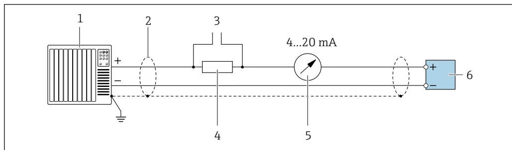
18 Пример подключения для токового выхода 4...20 мА HART (активного)
