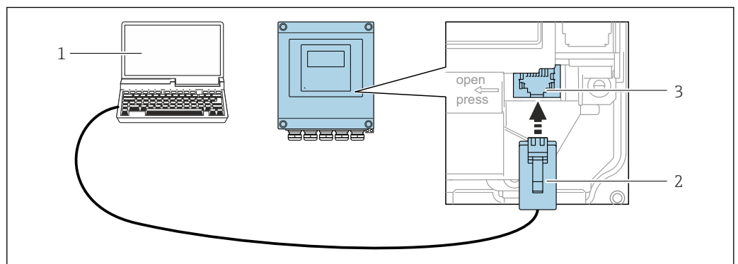
34 Подключение через служебный интерфейс (CDI-RJ45)
