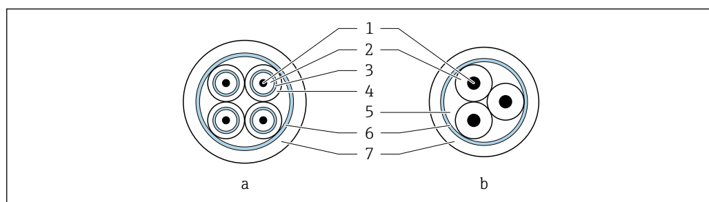
15 Поперечное сечение кабеля
