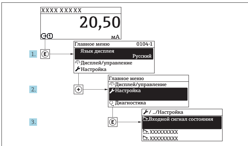
37 Пример индикации на локальном дисплее
