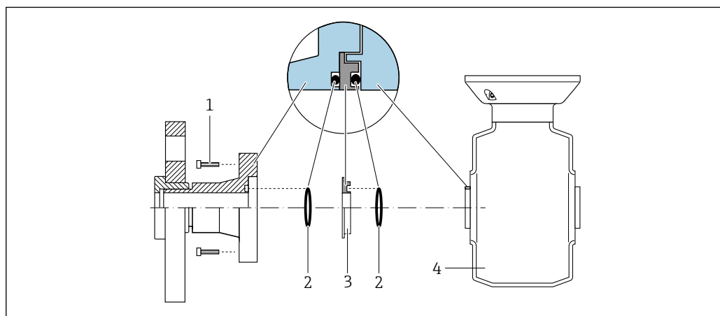
10 Установка колец заземления
