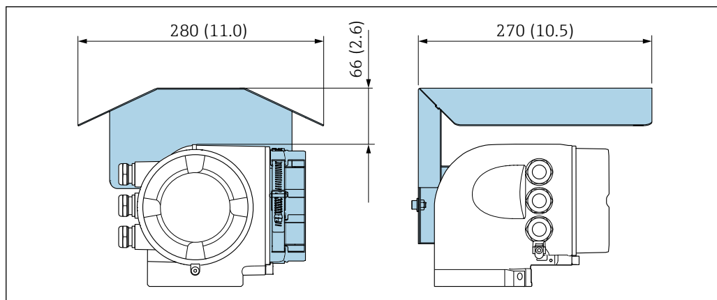
9 Защитный козырек от атмосферных явлений для Proline 500
