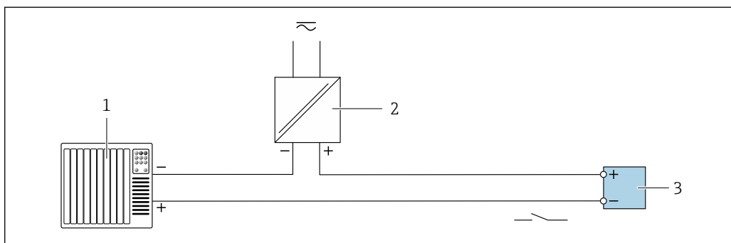
29 Пример подключения релейного выхода (пассивного)
