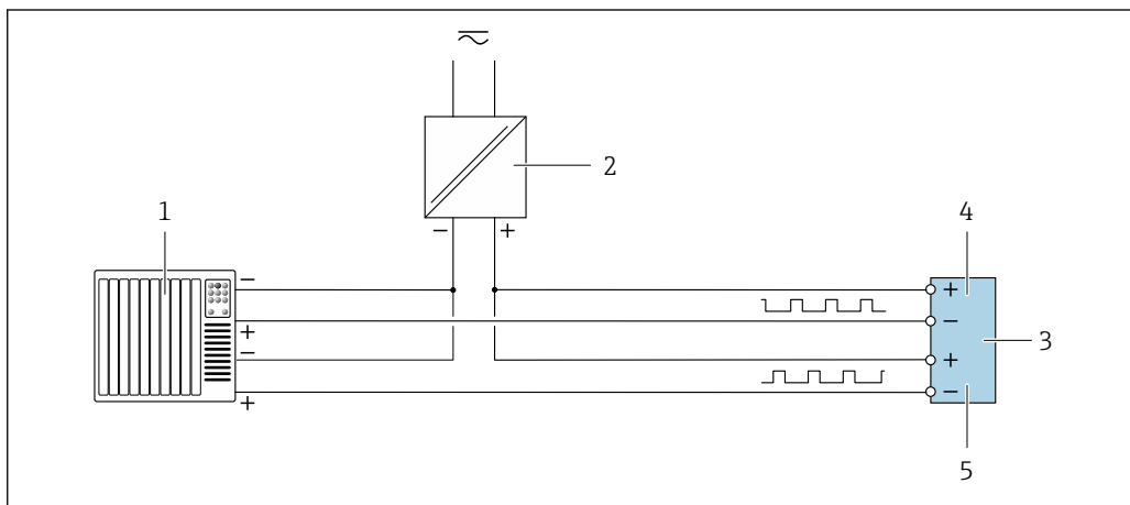
28 Пример подключения двойного импульсного выхода (пассивного)
