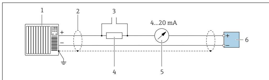
20 Пример подключения для токового выхода 4...20 мА HART (активного)
