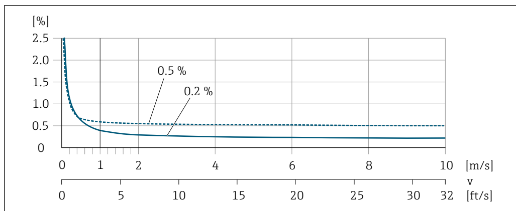
46 Максимальная погрешность измерения в % ИЗМ
